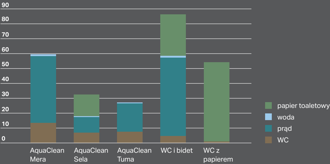
PORÓWNANIE TOALET MYJĄCYCH GEBERIT AQUACLEAN Z KONWENCJONALNYMI MISKAMI, W KTÓRYCH KORZYSTA SIĘ Z PAPIERU TOALETOWEGO, ORAZ Z BIDETAMI
